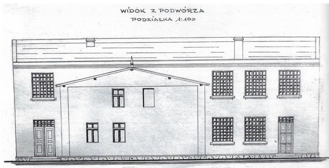
Ilustr. 99. Dom Rzemieśniczy w Potulicach. Rysunek pt. „Widok z podwórza. Podziałka 1:100”, ilustrujący widok z podwórza przebudowywanej w Potulicach cieplarni na warsztaty. Rysunek sporządzony w sierpniu 1934 roku przez kierownika budowy Franciszka Ossowskiego z Nakła. Skan (kopia) został wykonany z dokumentów znajdujących się w zasobach Archiwum Państwowego w Bydgoszczy
