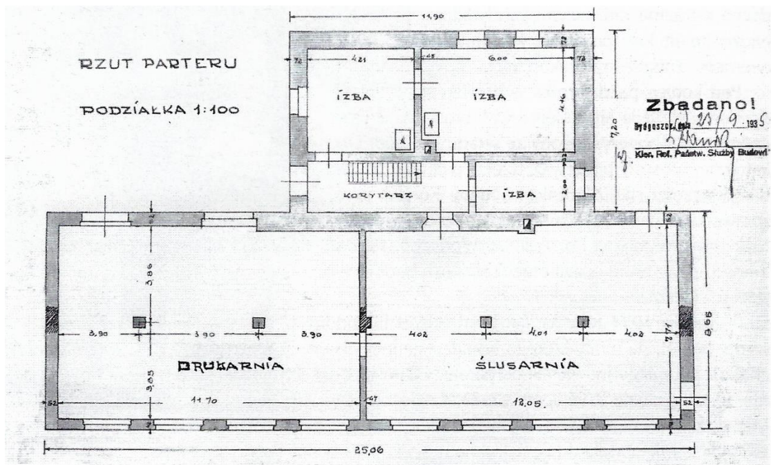
Ilustr. 100. Dom Rzemieślniczy w Potulicach. Rysunek pt. „Rzut parteru przebudowywanej w Potulicach cieplarni na warsztaty”. Rysunek sporządzony przez kierownika budowy Franciszka Ossowskiego z Nakła. Skan (kopia) został wykonany z dokumentów znajdujących się w zasobach Archiwum Państwowego w Bydgoszczy
