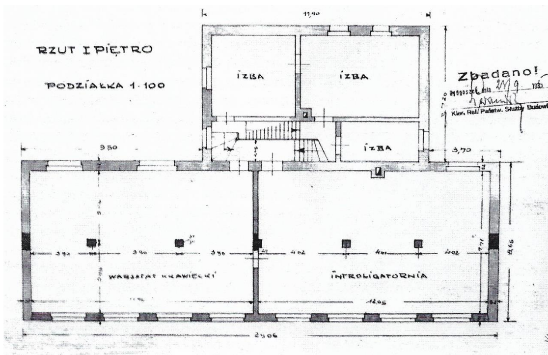
Ilustr. 101. Dom Rzemieślniczy w Potulicach. Rysunek pt. „Rzut piętra przebudowywanej w Potulicach ciepłarni na warsztaty”. Rysunek sporządzony przez kierownika budowy Franciszka Ossowskiego z Nakła. Skan (kopia) został wykonany z dokumentów znajdujących się w zasobach Archiwum Państwowego w Bydgoszczy
